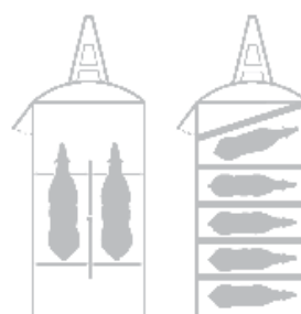
Typiska uppdelningslayouter HB610
